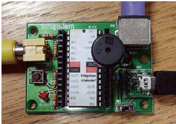
マイコンボード「IchigoJam」
