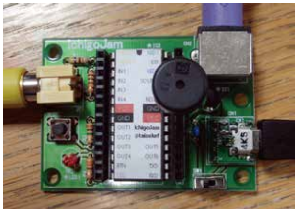
組み立てた「IchigoJam」
